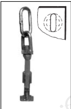
Drehschlüssel mit Sicherung Best.-Nr.: 2-7-WZ/DS Preis: 99,00 € pro Stück
