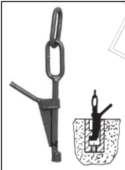
Schlüssel mit Keil Best.-Nr.: 2-7-WZ/SK
